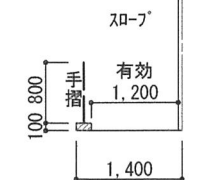
【立ち上がり部断面図】
