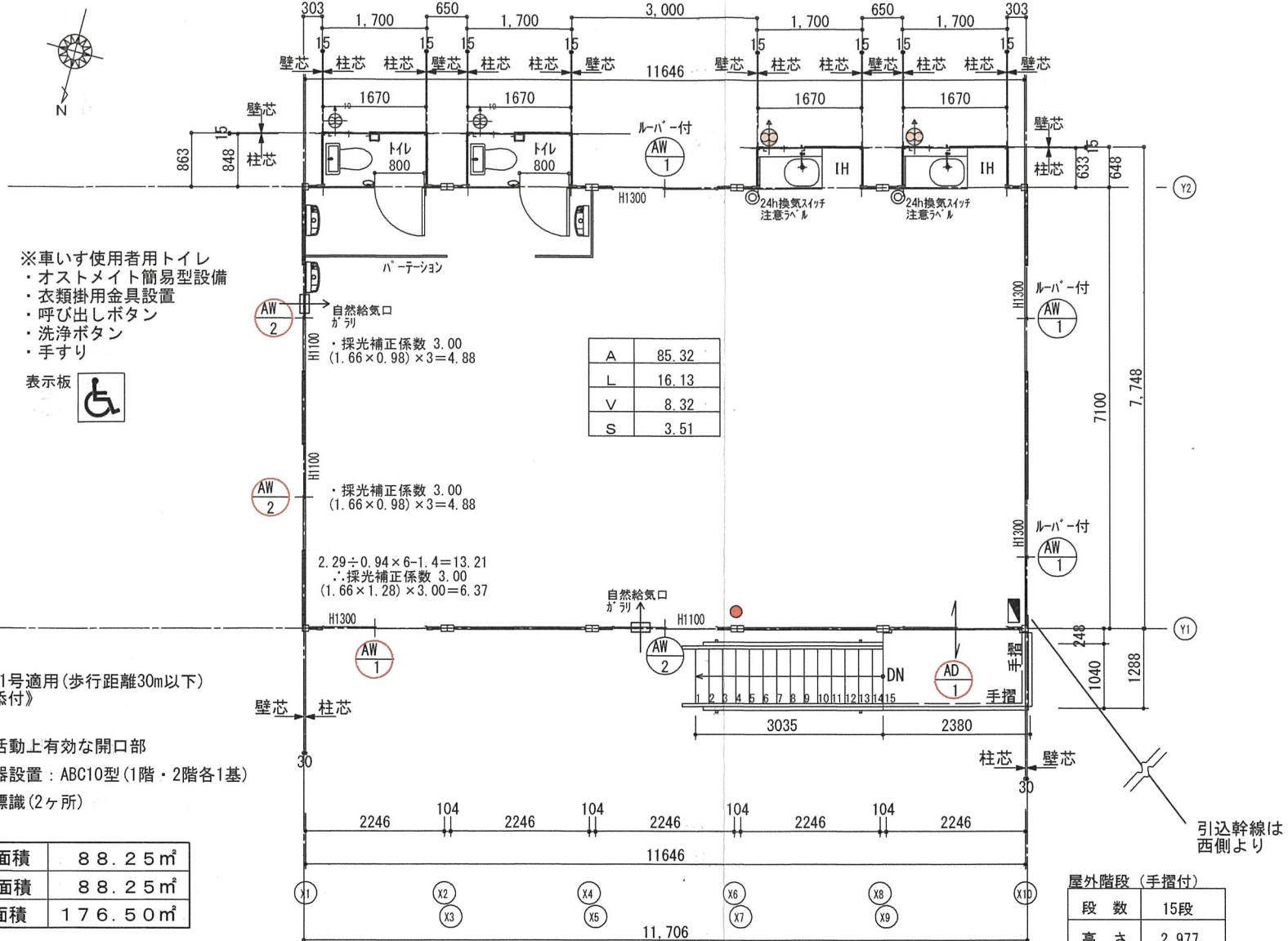
2階平面図
