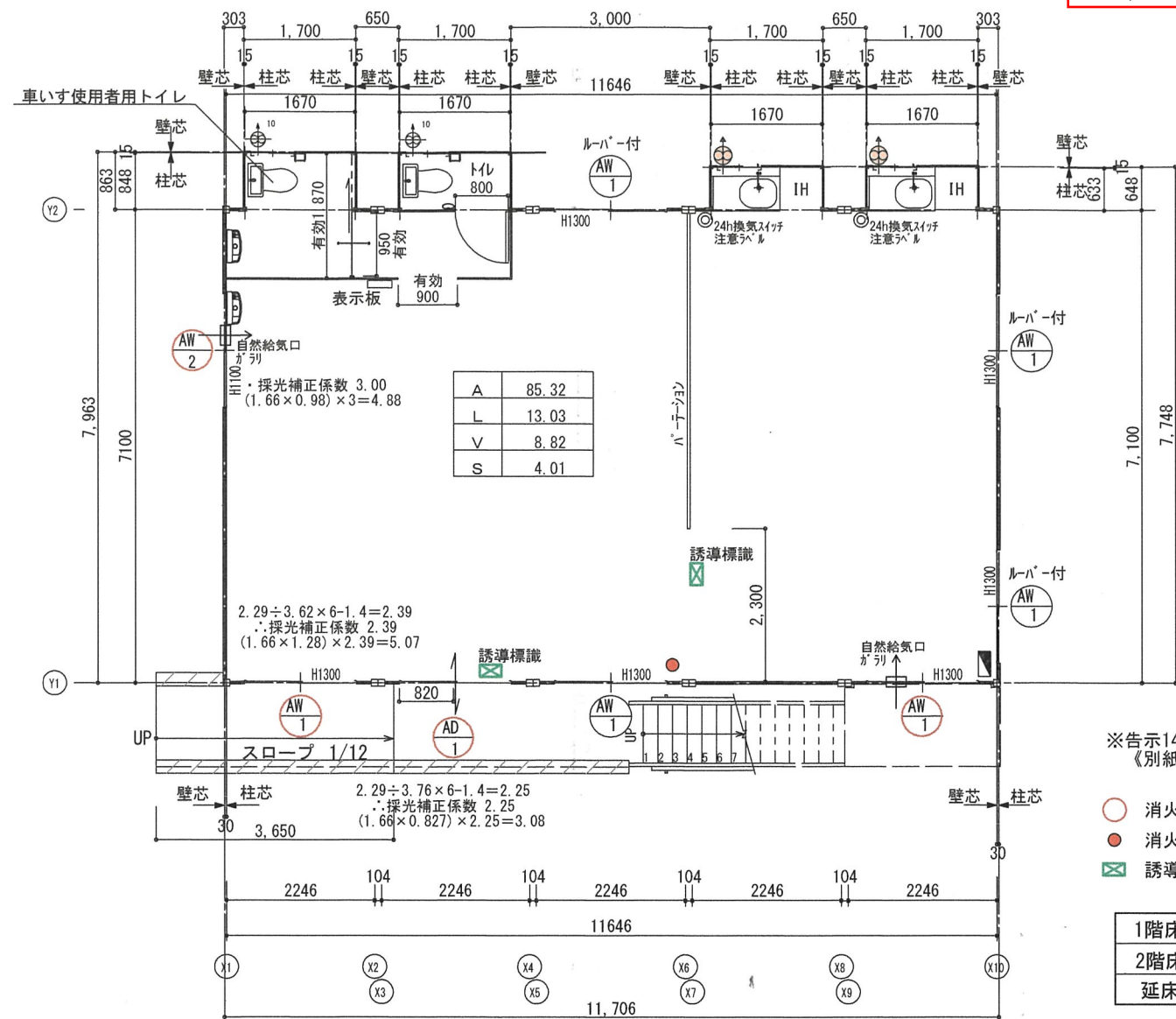
1階平面図
