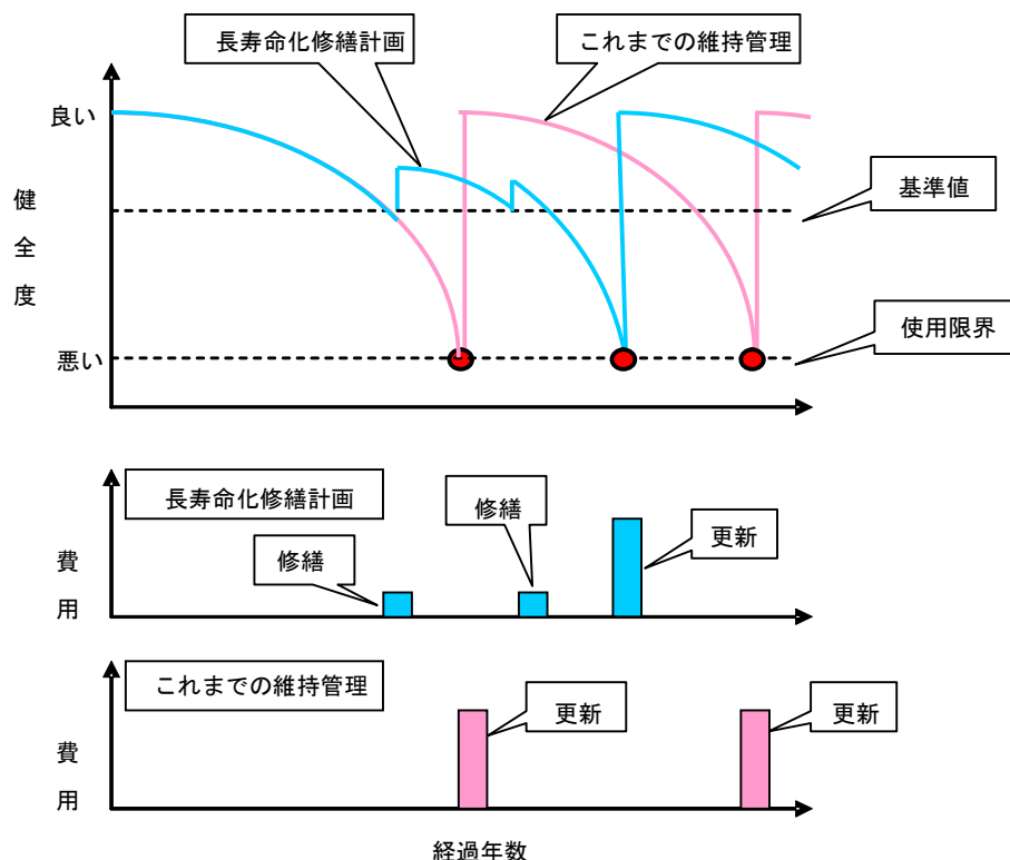
これまでの維持管理（事後対応型）と長寿命化修繕計画（予防保全型）の更新及び劣化イメージ図
