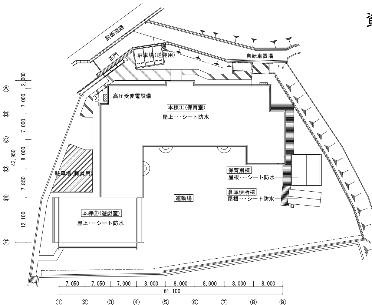
西保育所配置図(改修後)
