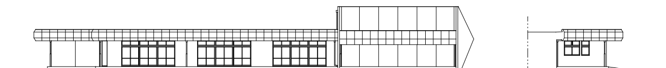
西側立面図(1)
