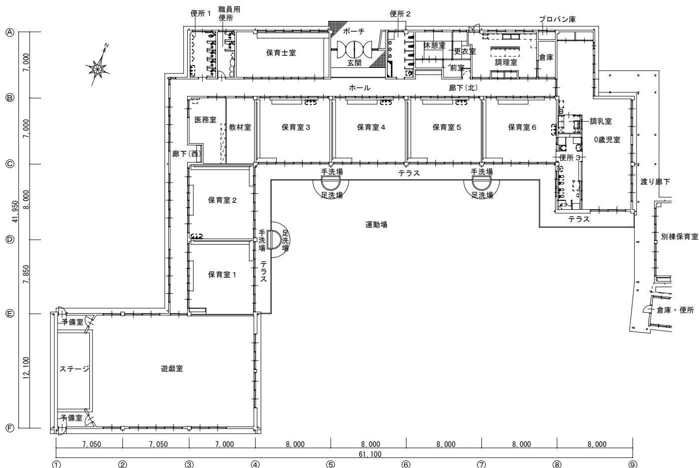
西保育所 平面図 (改修前)
