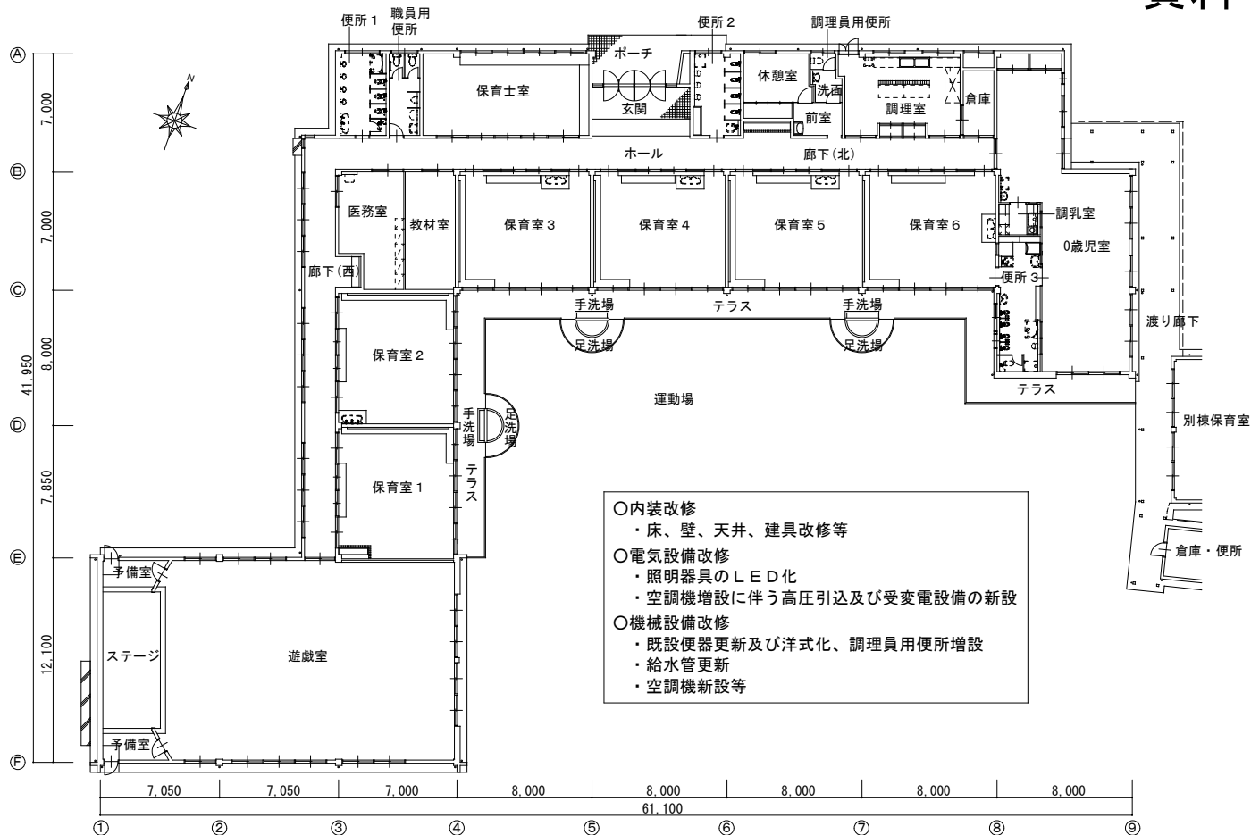
西保育所 平面図 (改修後)
