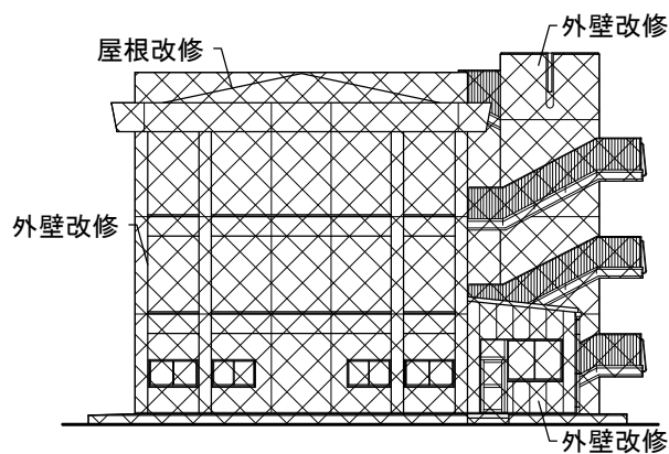
東立面图
