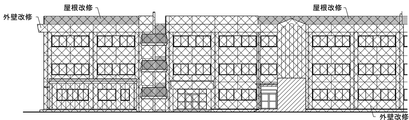
北立面图
