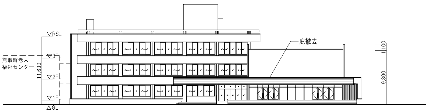
南立面図
