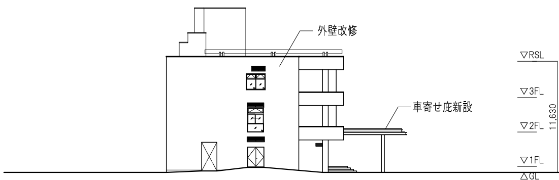
西立面図
