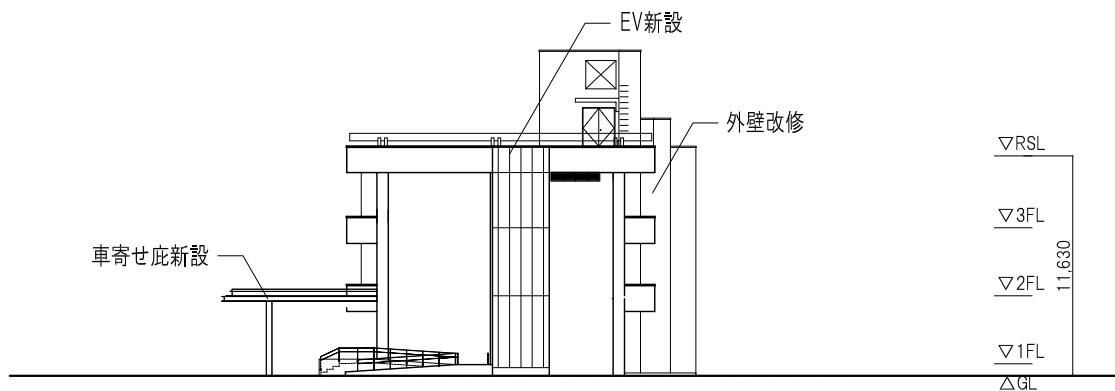
東立面図
