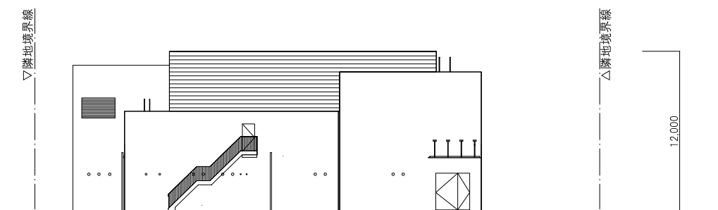
南立面図
