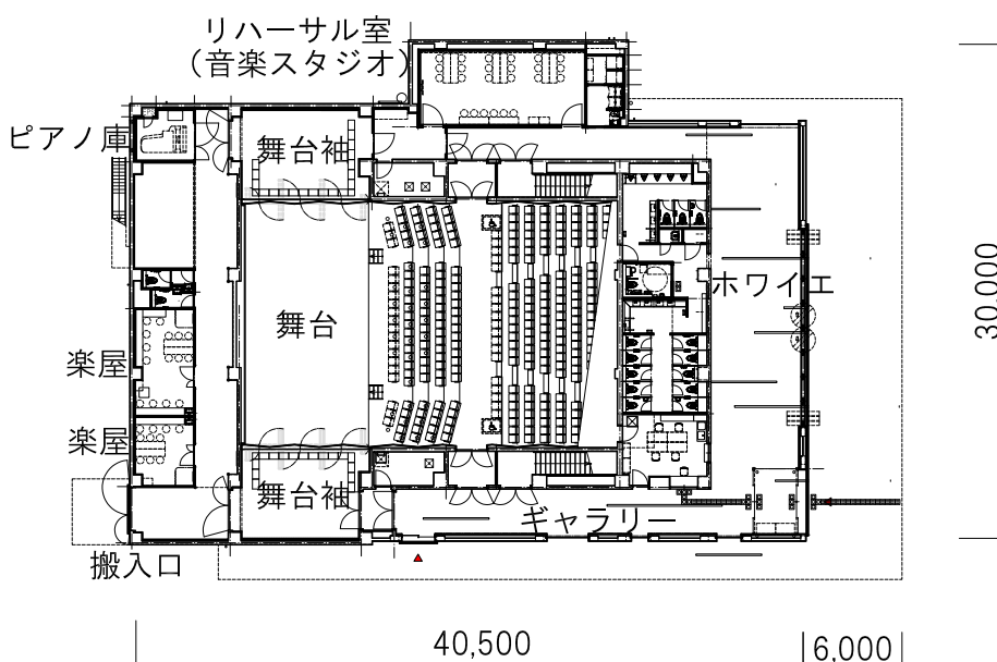
1階平面図
