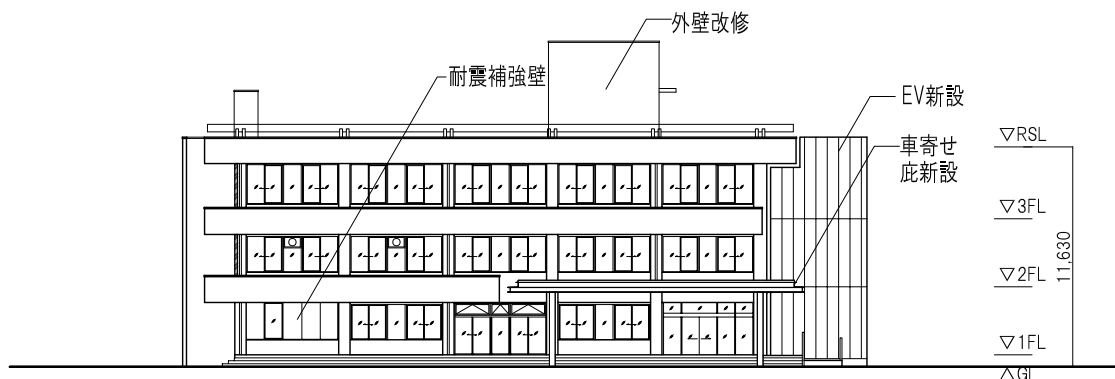
南立面図
