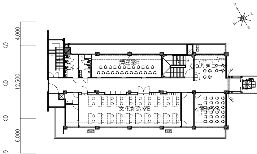
3階平面図
