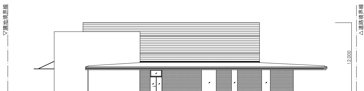
東立面図
