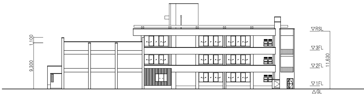
北立面図
