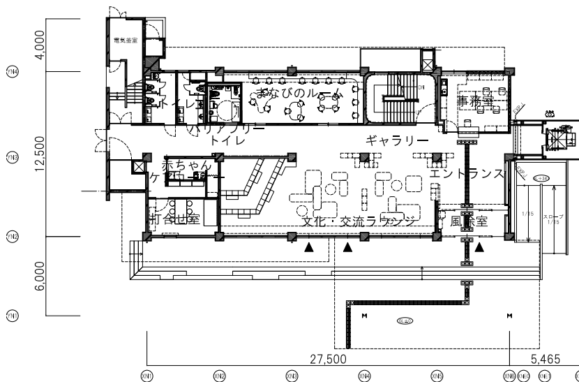
2階平面図
