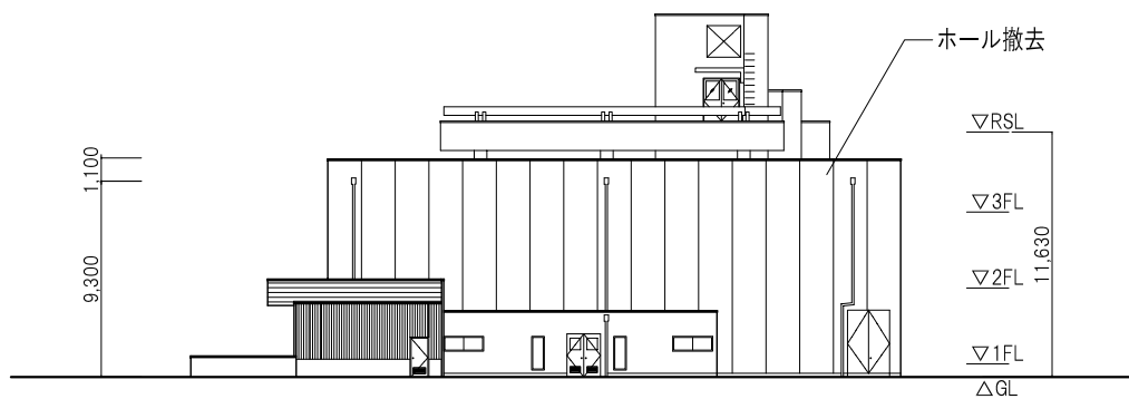
東立面図
