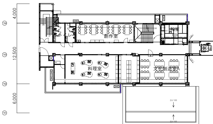
2階平面図
