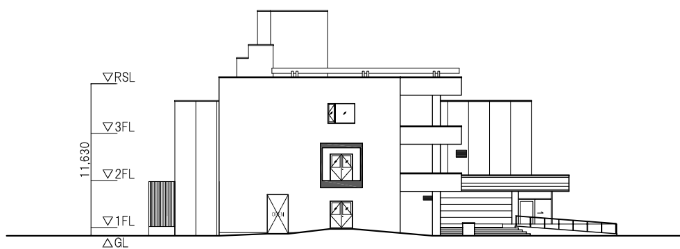
西立面図
