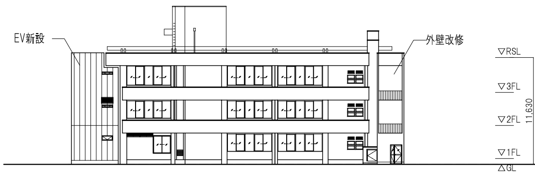
北立面図
