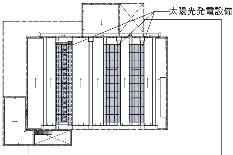
屋上平面図
