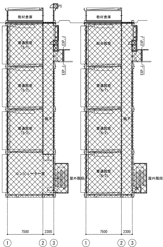
2階平面図
