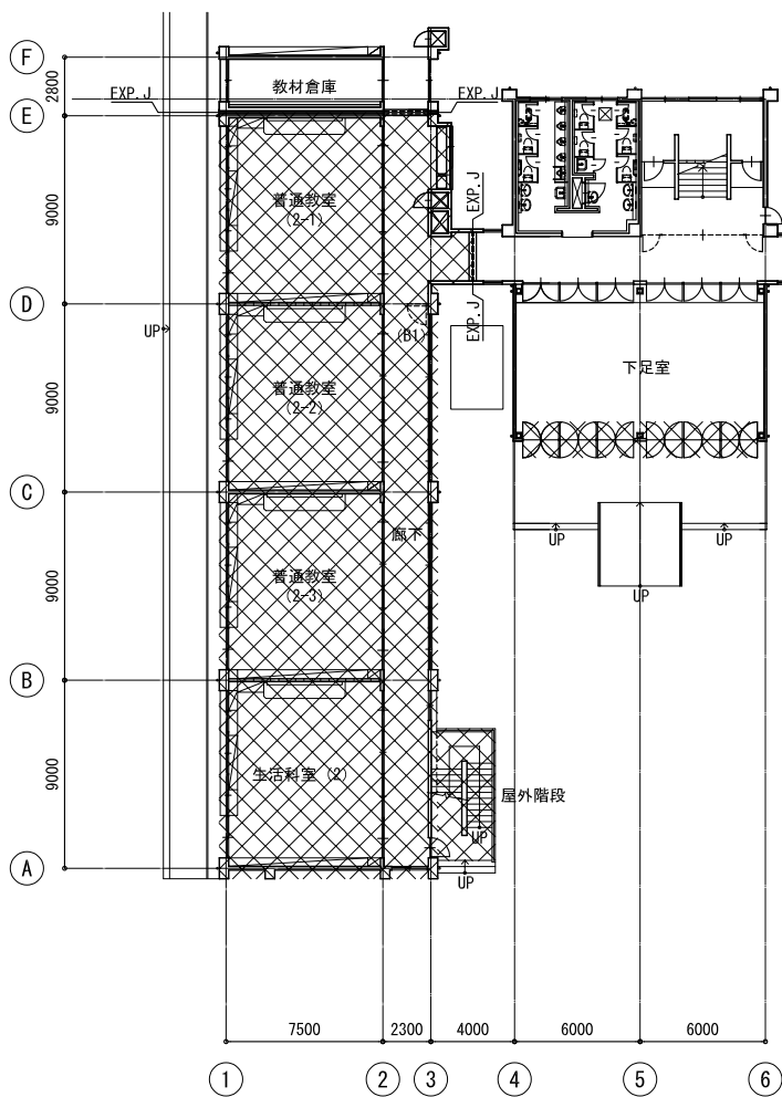
1階平面図
