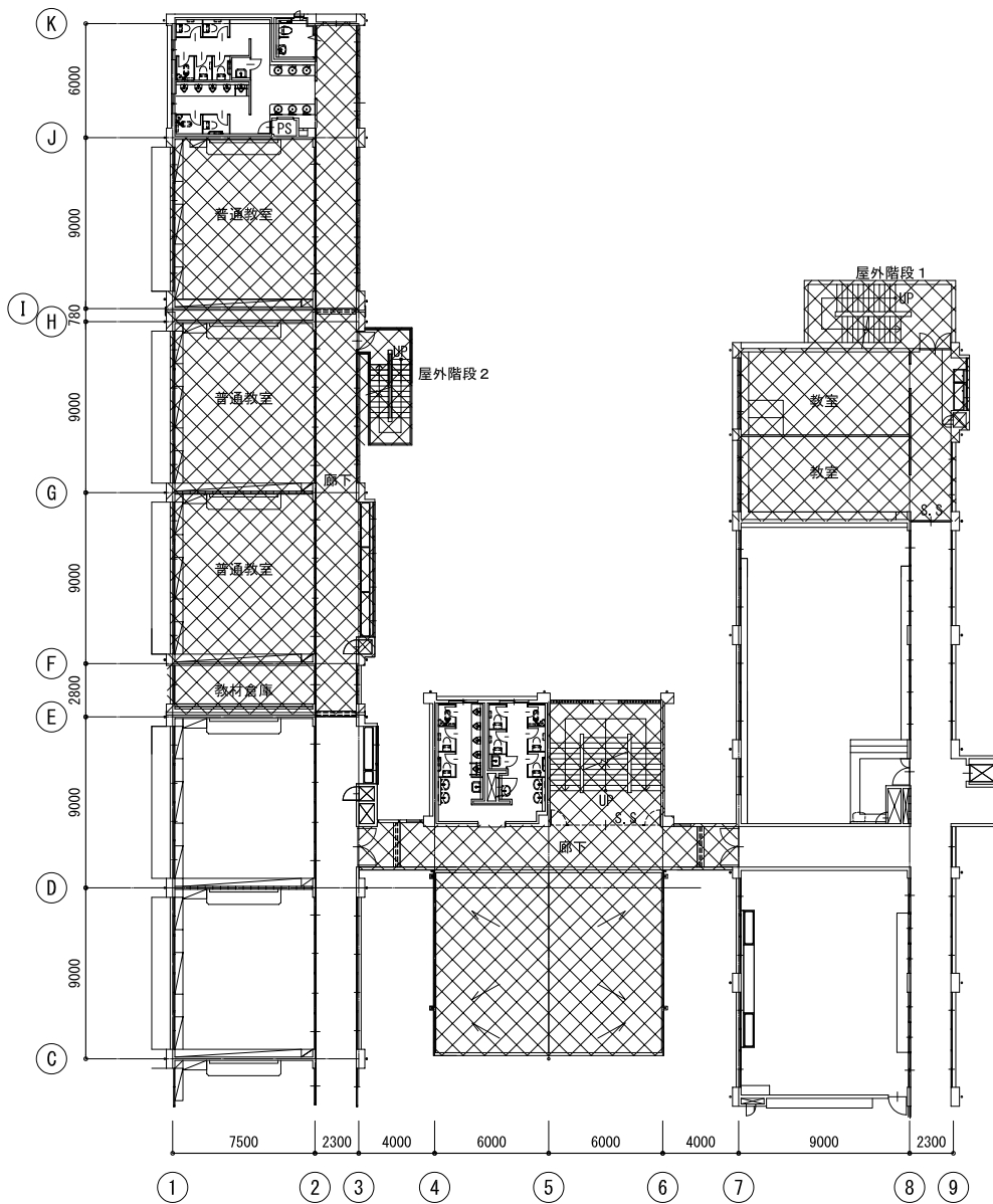
2階平面図
