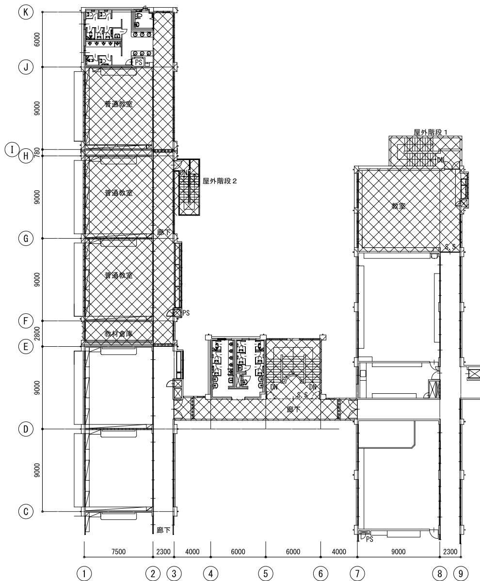
3階平面図
