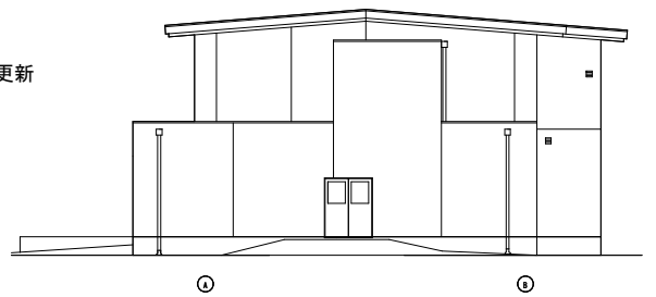
東立面図
