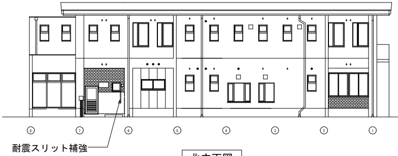
北立面図
