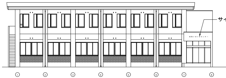
南立面図
