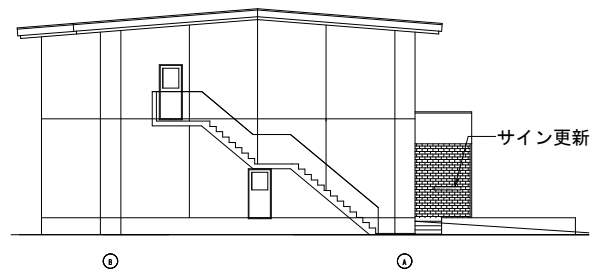
西立面図
